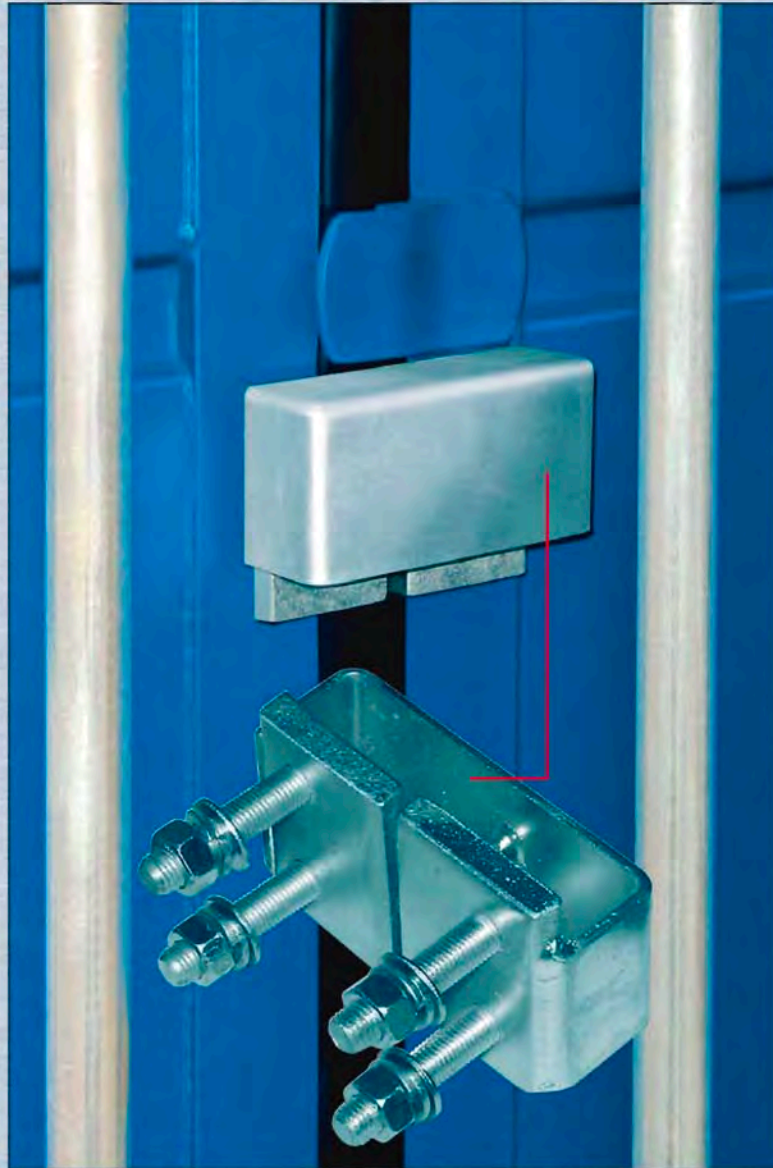
Portes de conteneur avec protection cadenas
