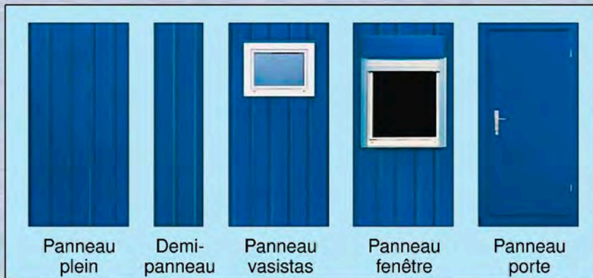
Le montage et le démontage des panneaux muraux peuvent être menés simplement et rapidement.
